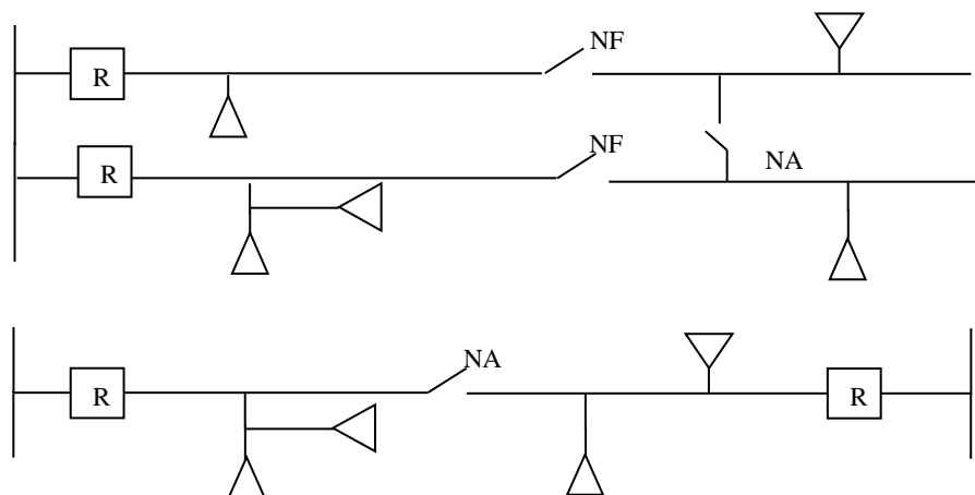
Figura 6 – Configuração Radial com Recurso
