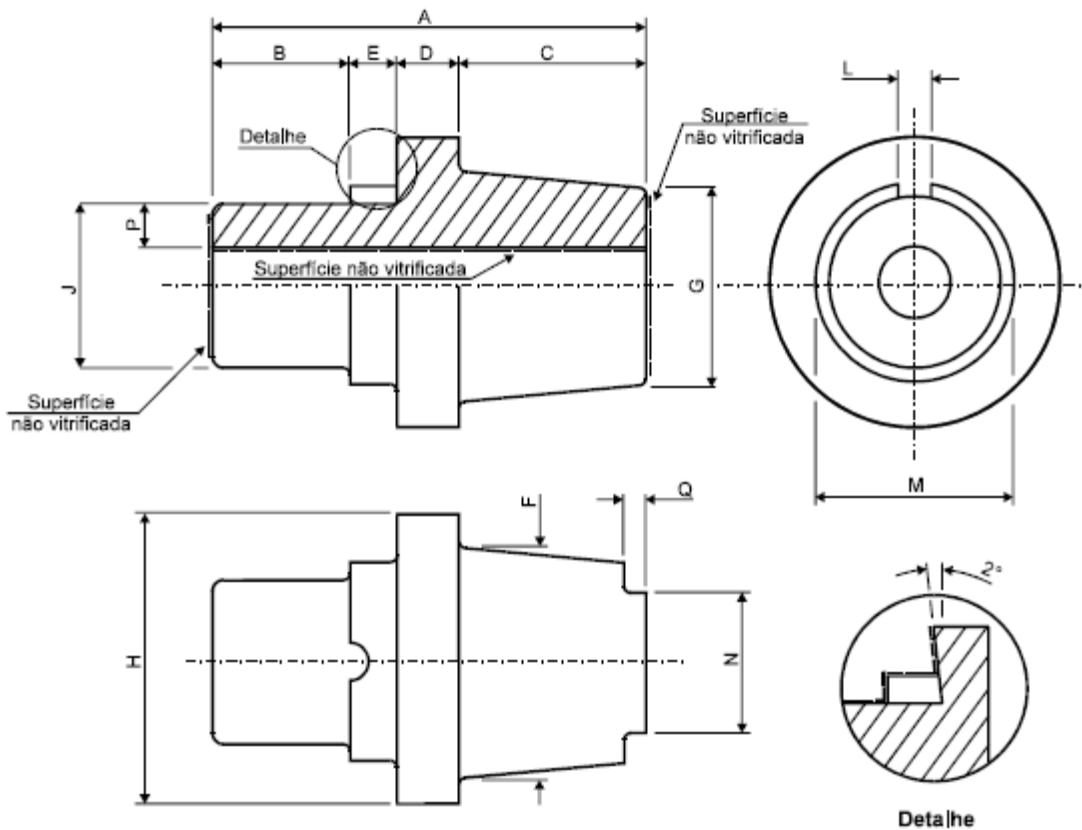
Figura 7 – Folha 5/6 - Bucha 1,3 kV - 160 A/400 A/800 A
