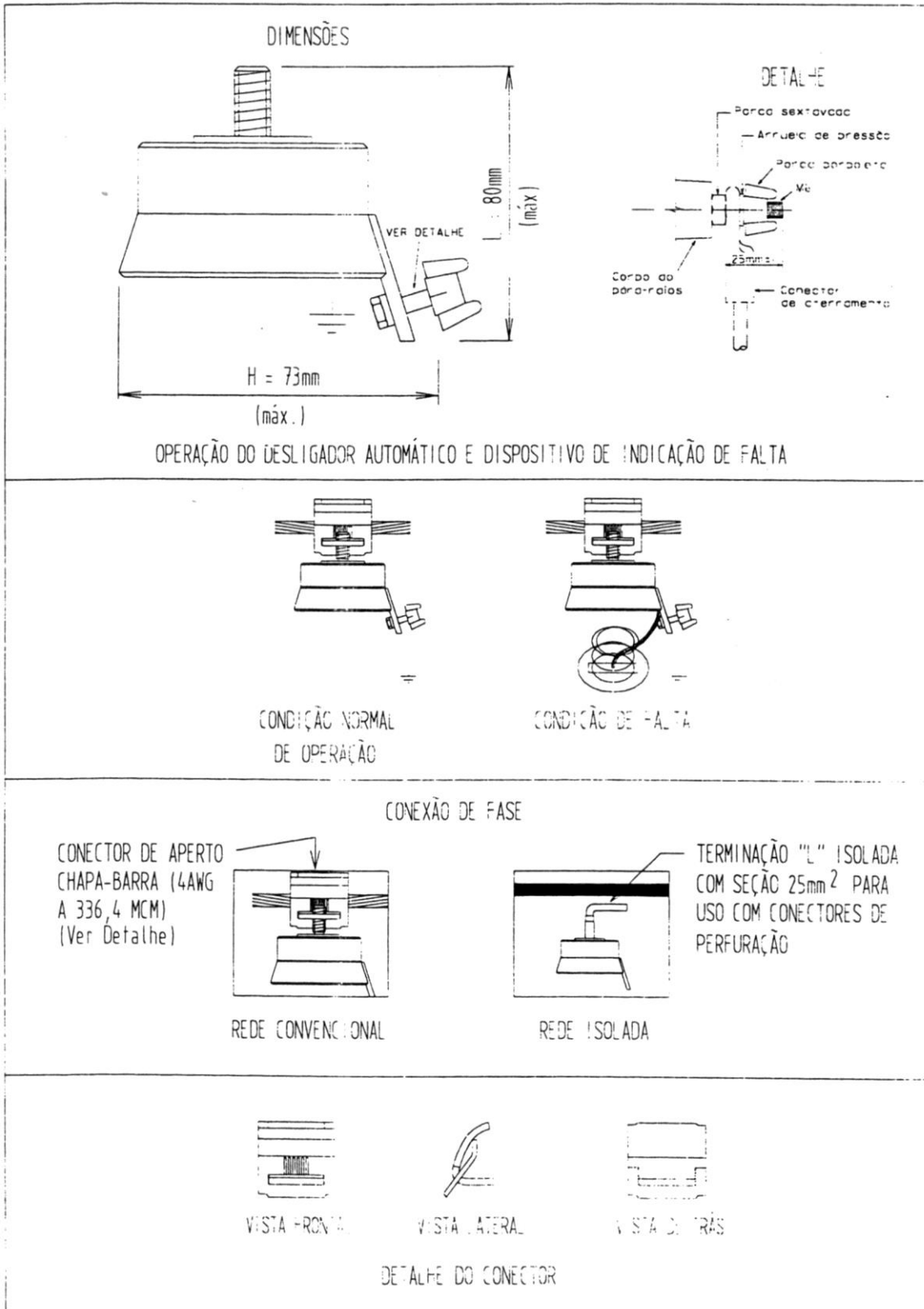
FIGURA 1 PARA-RAIOS DE BAIXA TENSÃO
