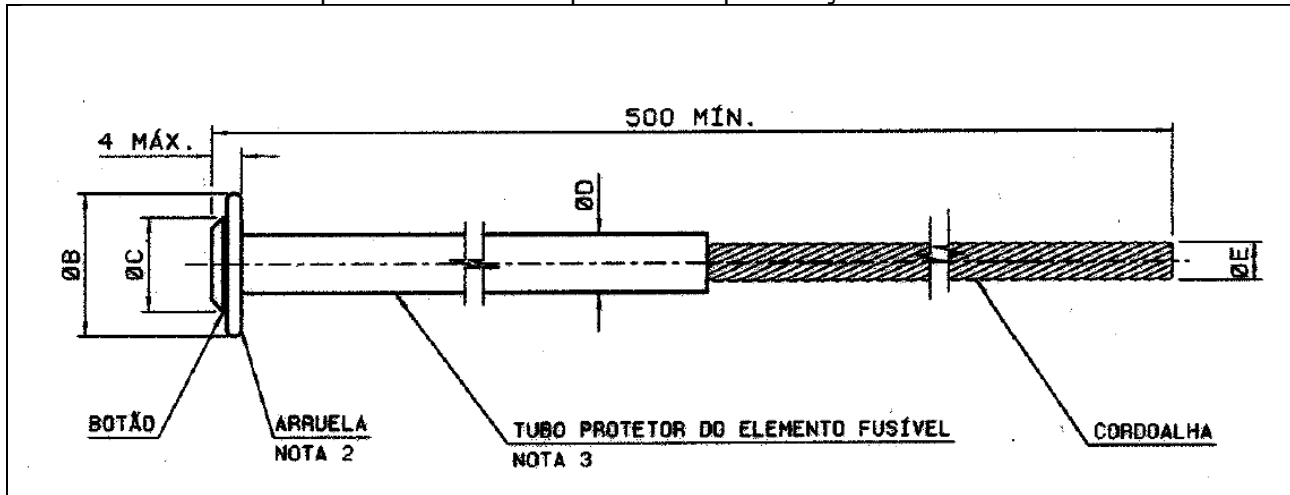
Figura 7 - Dimensões padronizadas e características dos fusíveis Unidades capacitivas cobertas por essa Especificação
