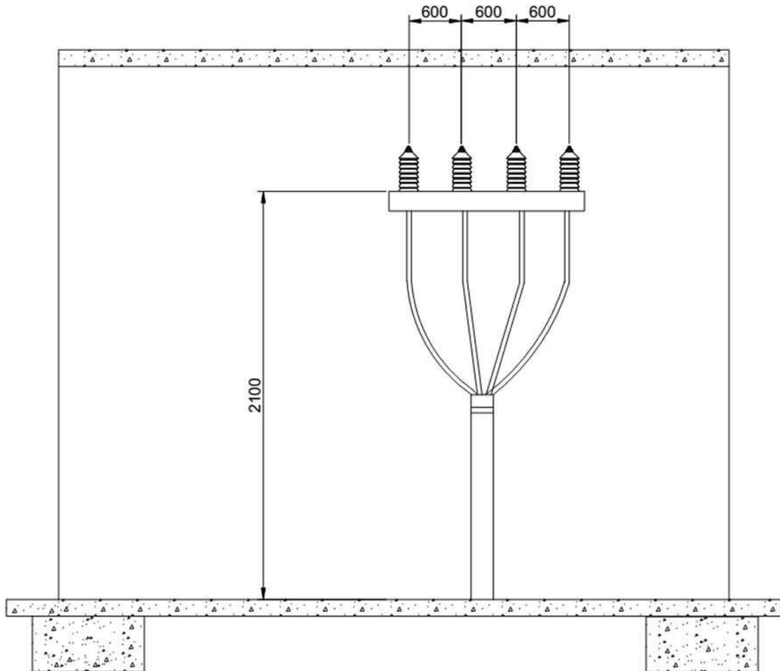
Detalhe da Mufra
