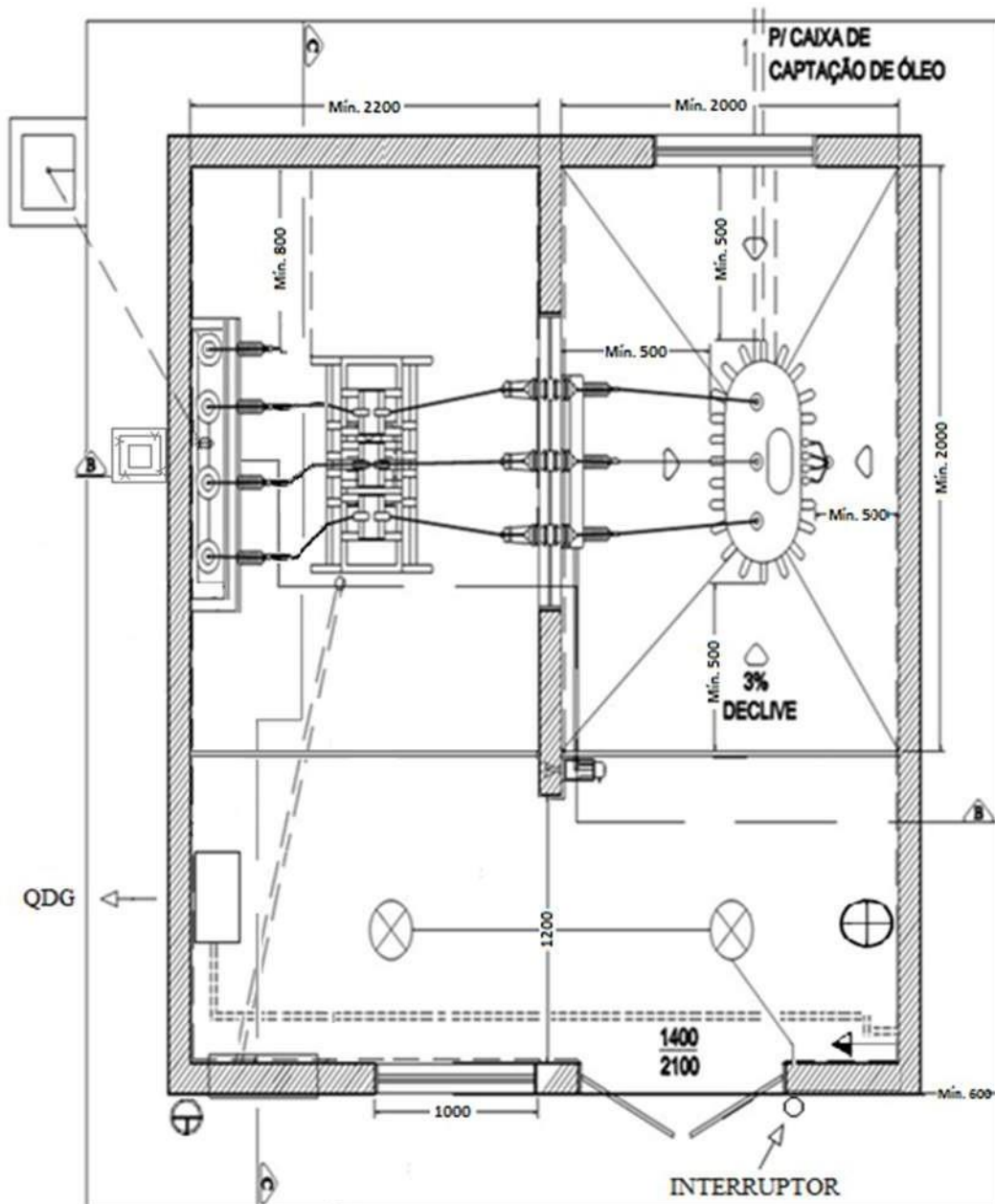
DESENHO 9 A – DETALHAMENTO SUBESTAÇÃO COM RAMAL DE LIGAÇÃO SUBTERRÂNEO
