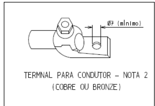
TERMINAL DE COBRE OU BRONZE PARA CONDUTOR (NOTA 2)
